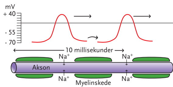
Figur 83. Nervesignalet.
